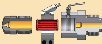
OFS-Filterdüse Typ SF „Einzelteile“
