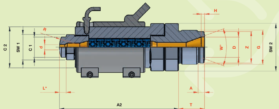
OFS-Mischdüse Typ XMD „Einzelteile“
