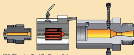
OFS-Filterdüse Typ UR „Einzelteile“
