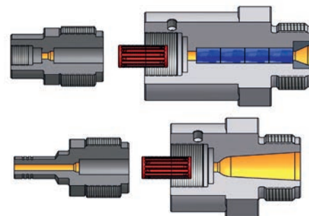
OFS-Filterdüse Typ SF optional mit Innengewinde, Mischeinsatz, Nadelsitz und Tauchansatz.
