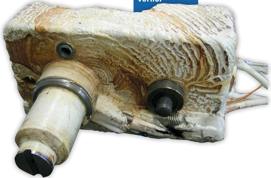
Heißkanalbalken vorher
